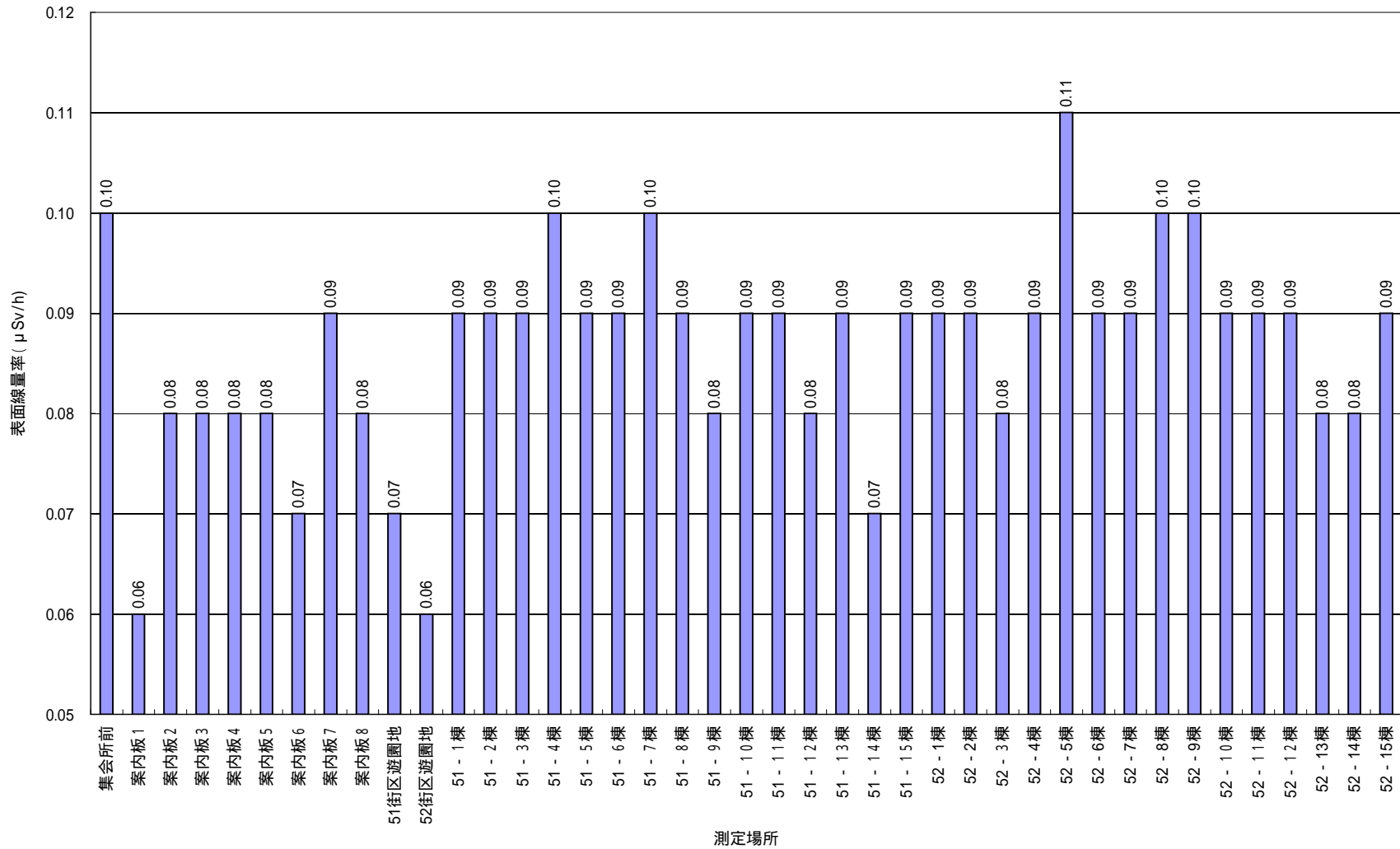
聖ヶ丘3丁目団地 地表面線量率 (μSv/h)測定結果 (2013年7月13日測定)
